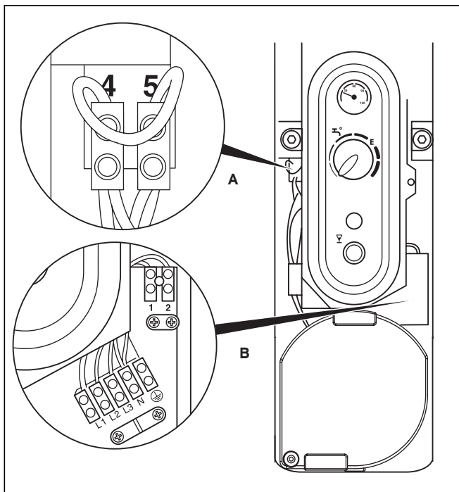
Рис. 8.5 Клеммная коробка
