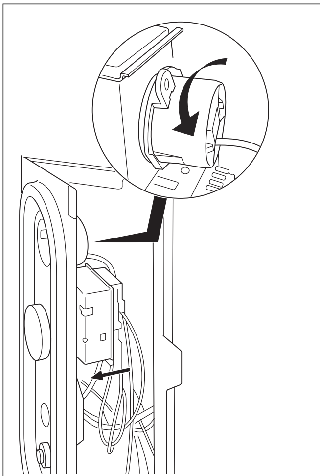
Рис. 7.13 Снятие термометра
