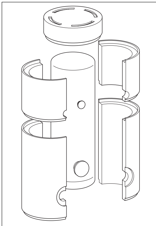
Рис. 7.18 Снятие изоляции
